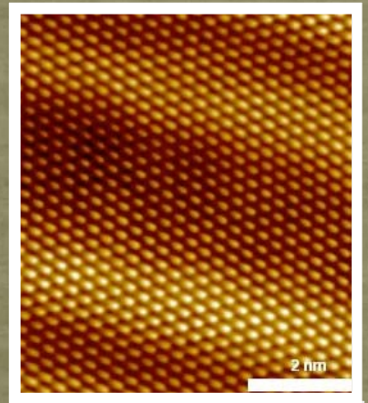
金原子結構
