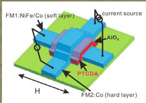
有機分子自旋閥
