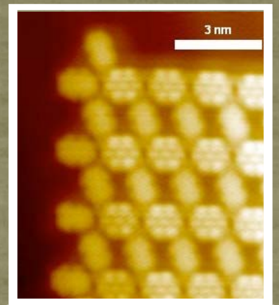
有機分子自組裝
