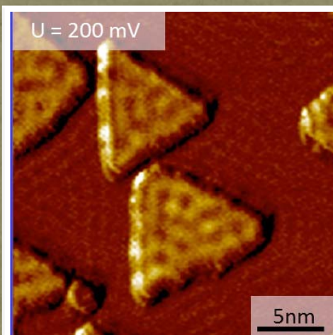
二維量子阱電子駐波
